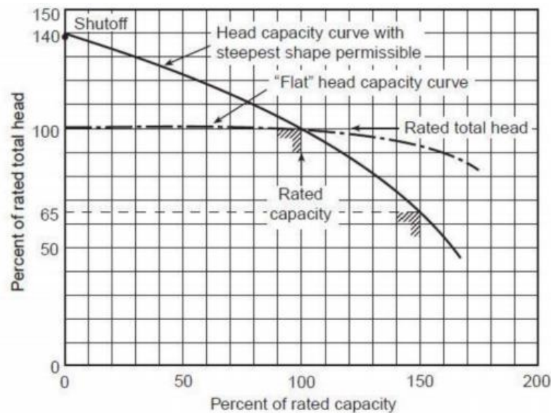
شکل ۶: منحنی عملکرد
